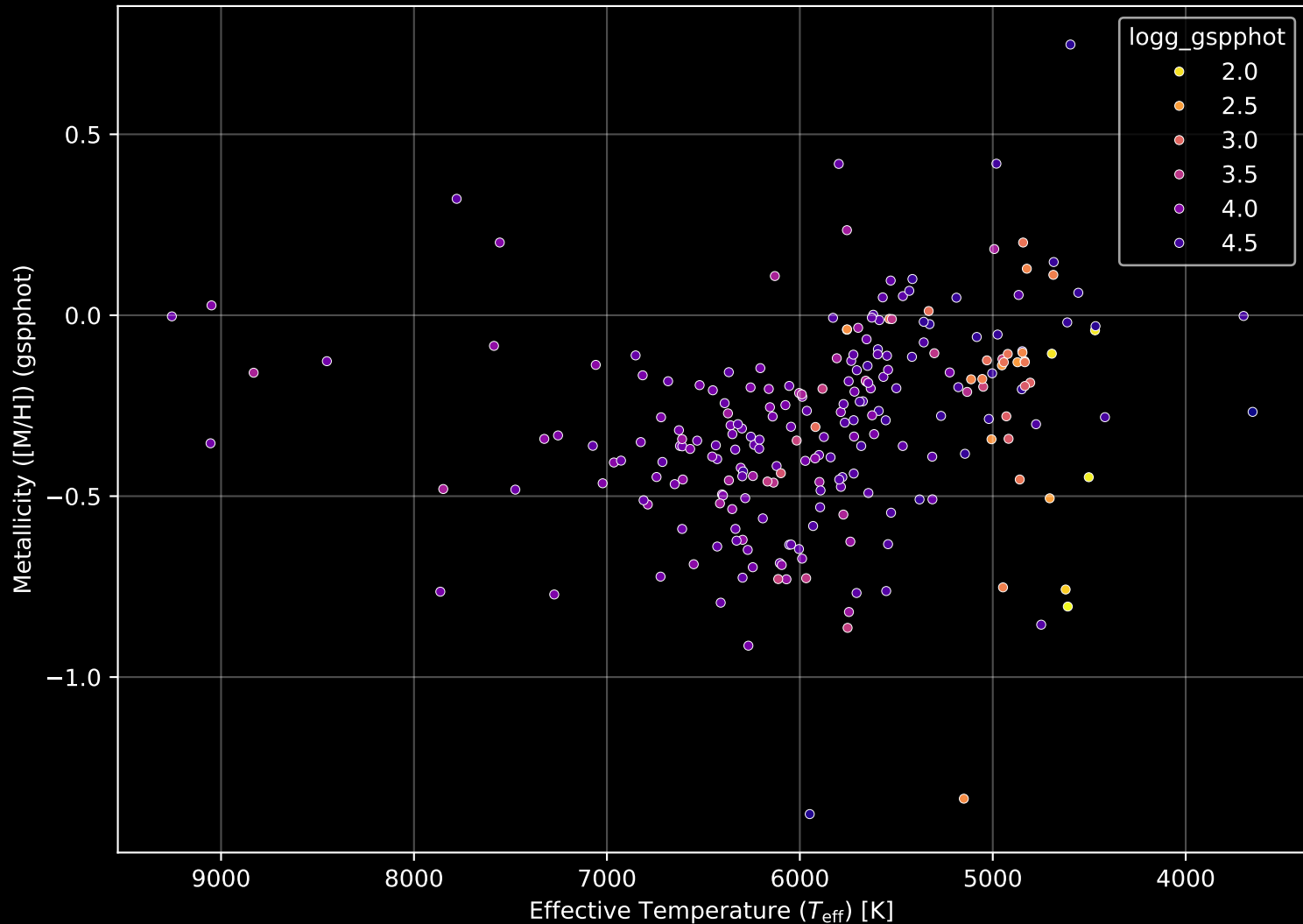
GALAH DR4 Field: [3168] Stellar Population Parameters (n= 238)
