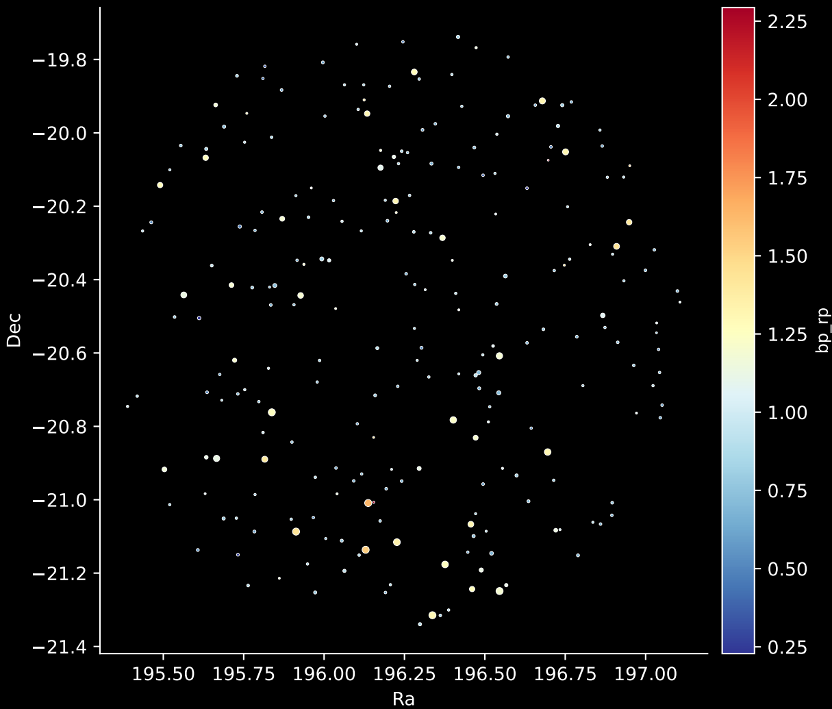
GALAH DR4 Field: [3168] Stars: 238
