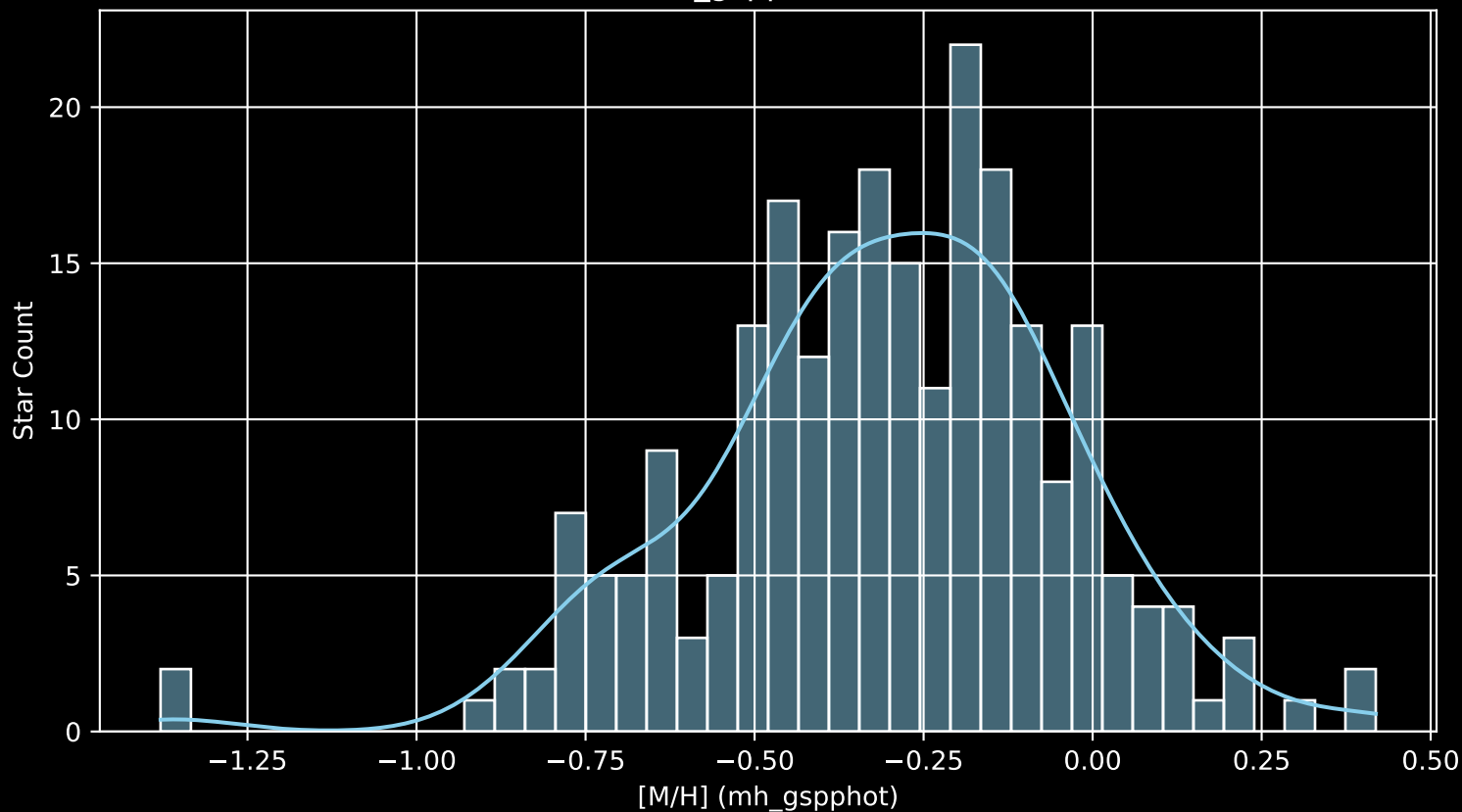
GALAH DR4 Field: [3168] [M/H] (mh_gspphot) (n= 237)
