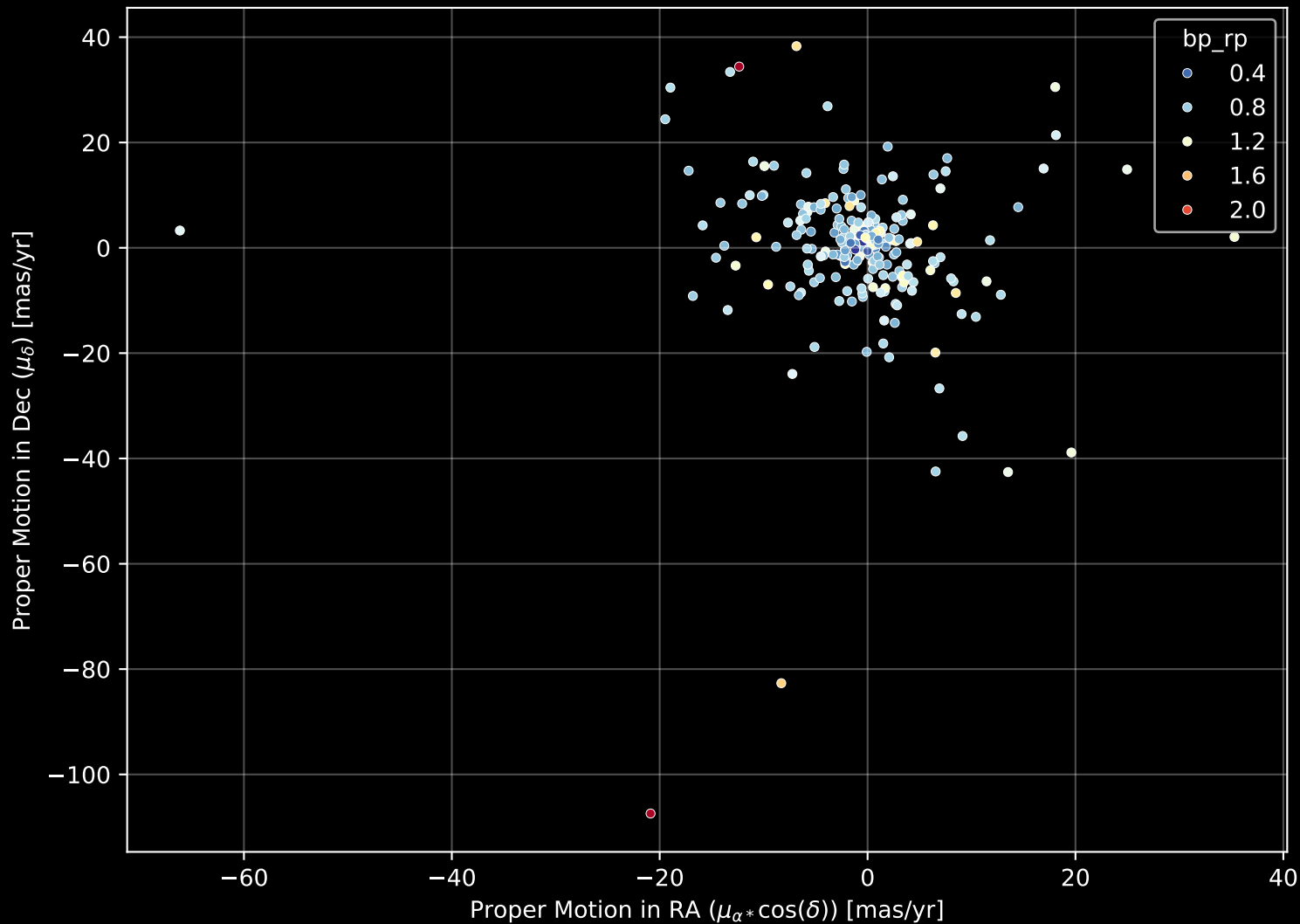
GALAH DR4 Field: [3168] Proper Motion Diagram (n= 238)
