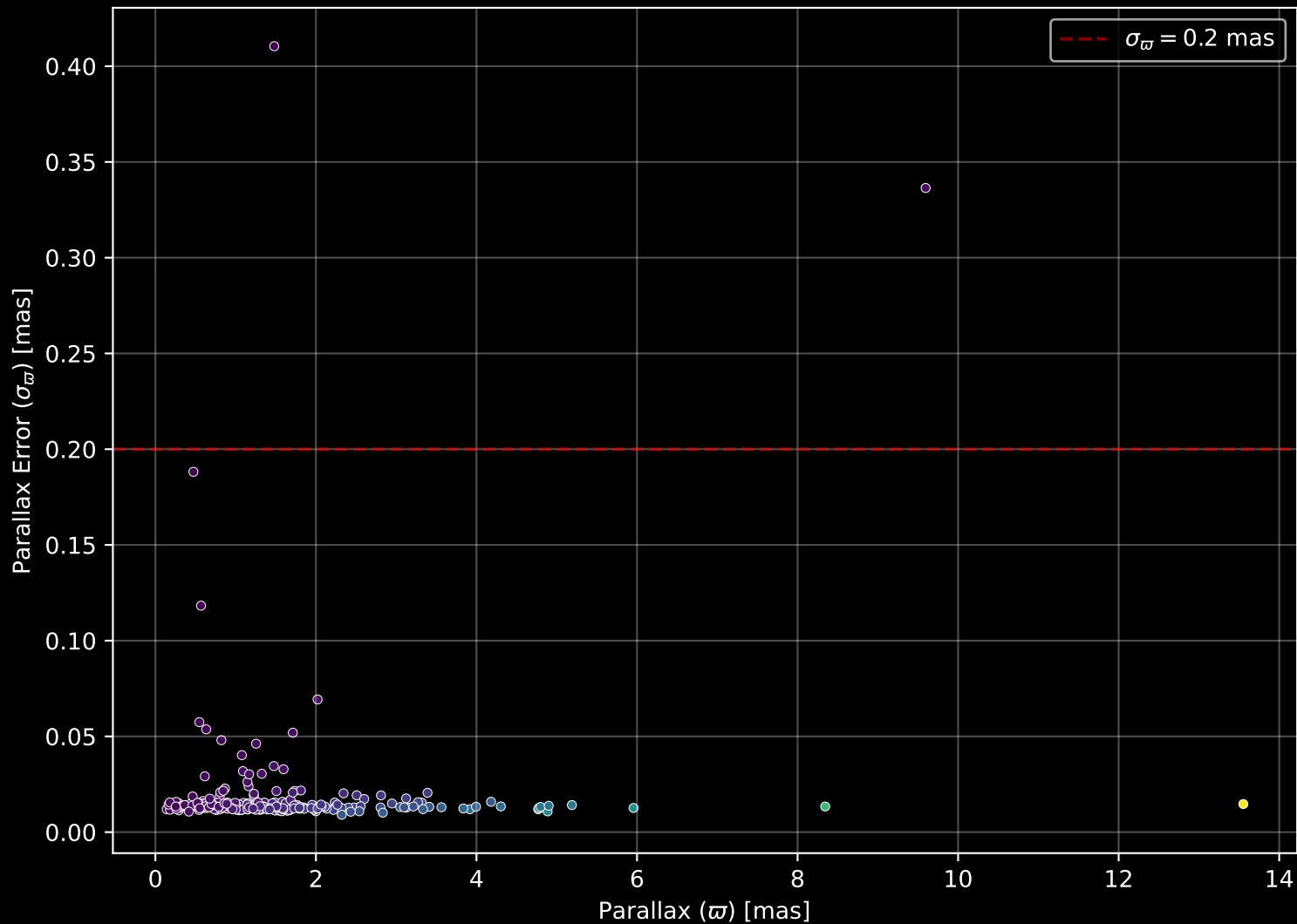
GALAH DR4 Field: [3168] Parallax Quality (n= 238)
